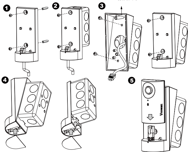
15° 倾斜支架
